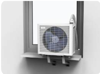
Coloque a unidade exterior no suporte
